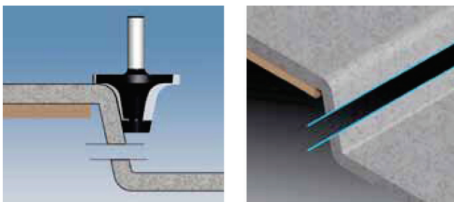
Фреза фасочна з опорним підшипником
