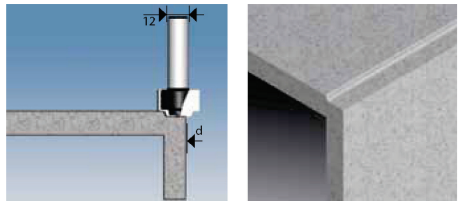
Фреза фасочна для ребер
