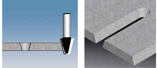
Фреза конусна 15° з нижньою ріжучою кромкою
