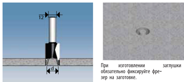
Фреза для виготовлення заглишок
