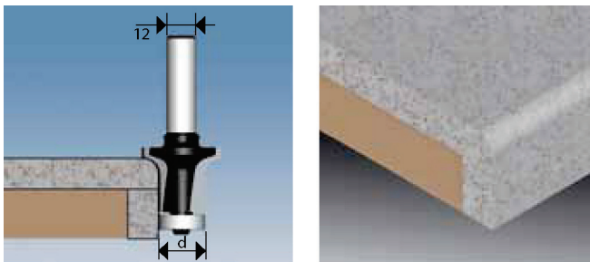
Фреза радіусна пригонююча з підшипником
