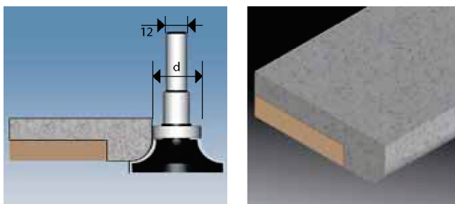
Фреза радіусна з верхнім підшипником
