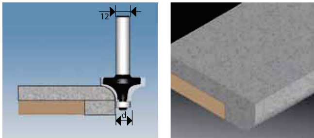
Фреза радіусна з нижнім підшипником
